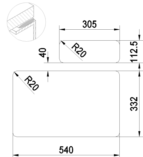
Einbau Unterbau Mounting base Montage de base Base de montaje
